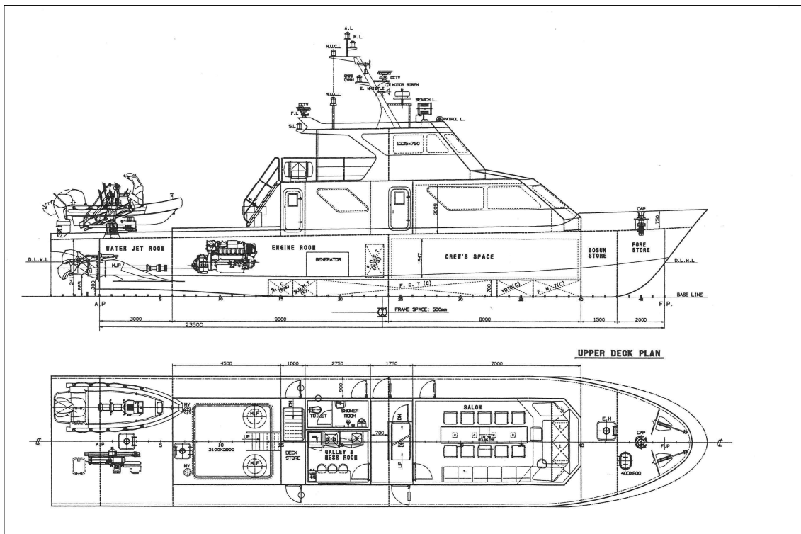
(어업지도선 설계도)
